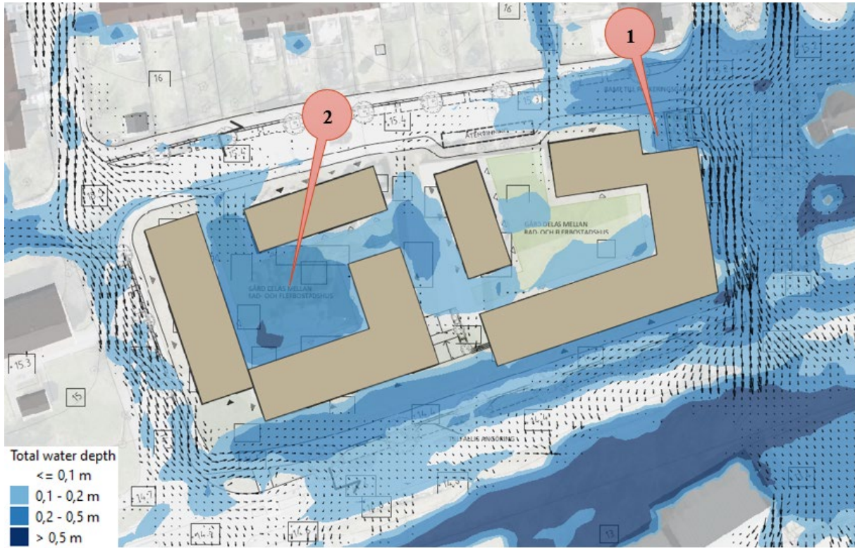
Figur 34: Skyfallssimulering med förslag 1
