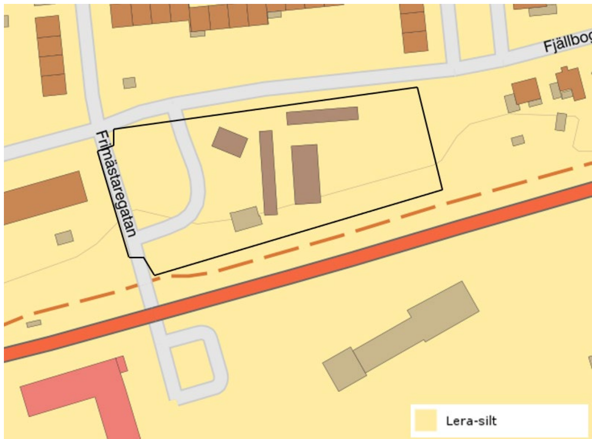
Figur 10. SGU:s jordartskarta. (SGU, 2022)
